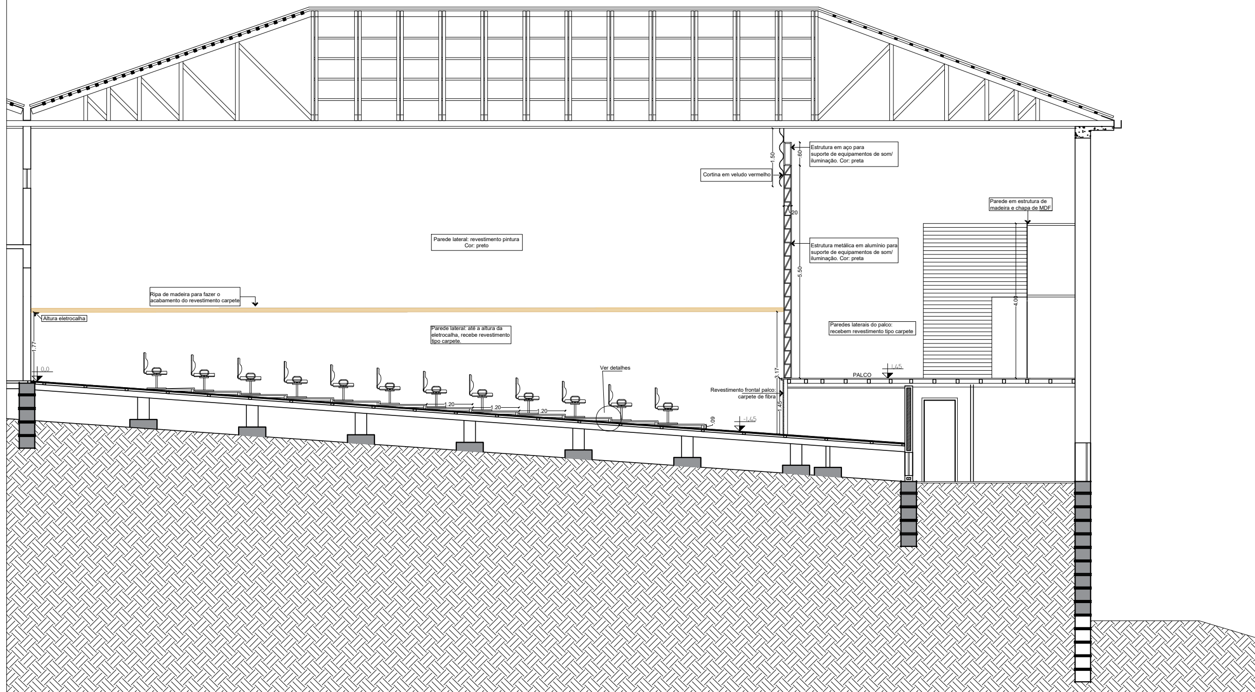
Vista/Corte — Esc.: 1/100
